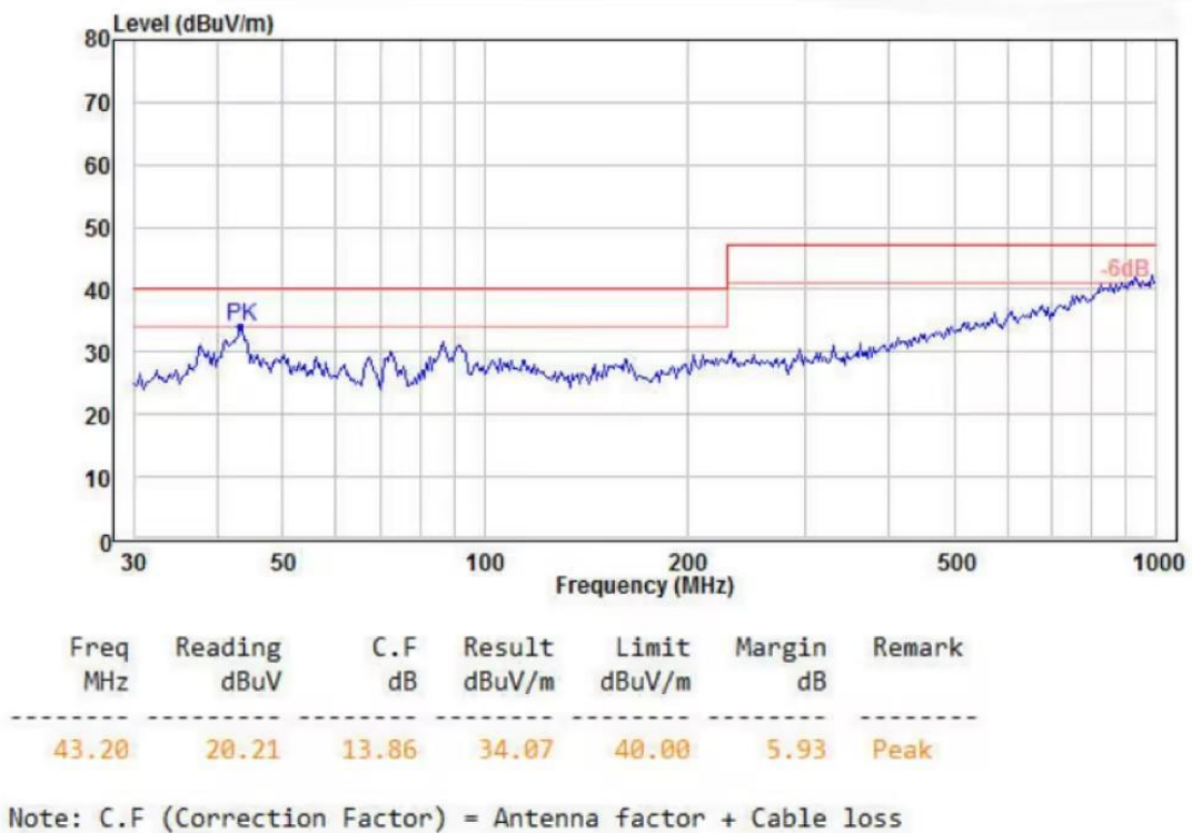
图 5-7 RE 测试垂直方向
