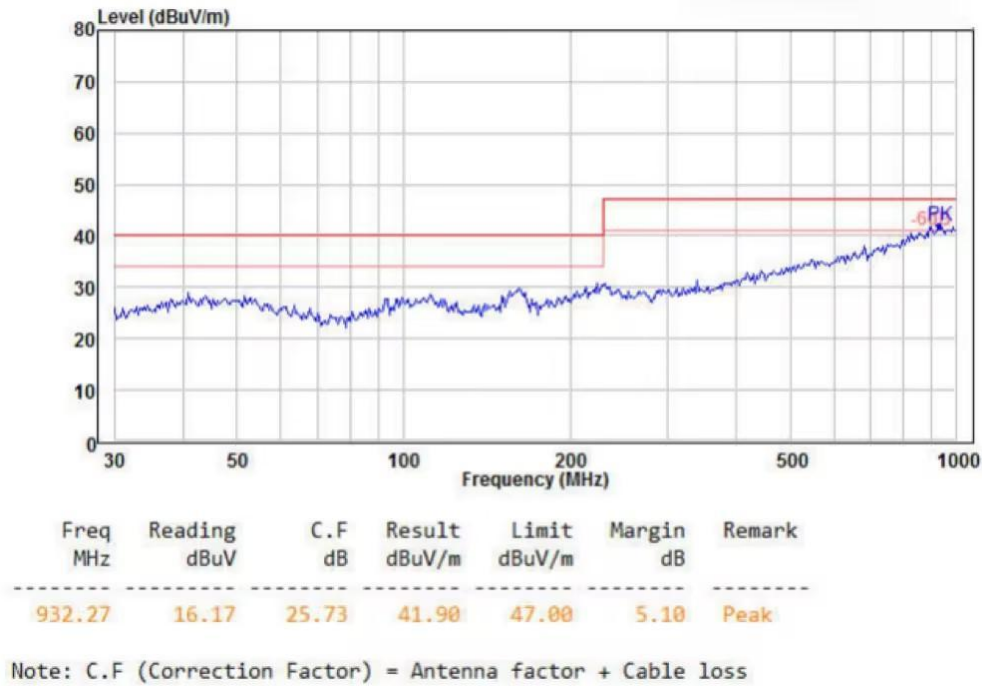
图 5-6 RE 测试水平方向
