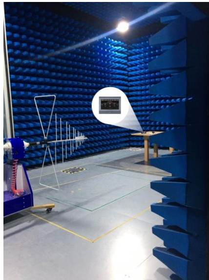
图 5-5 RE 测试图
