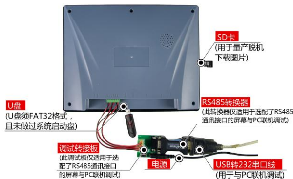
图 1-4 RS485 调试工具图
