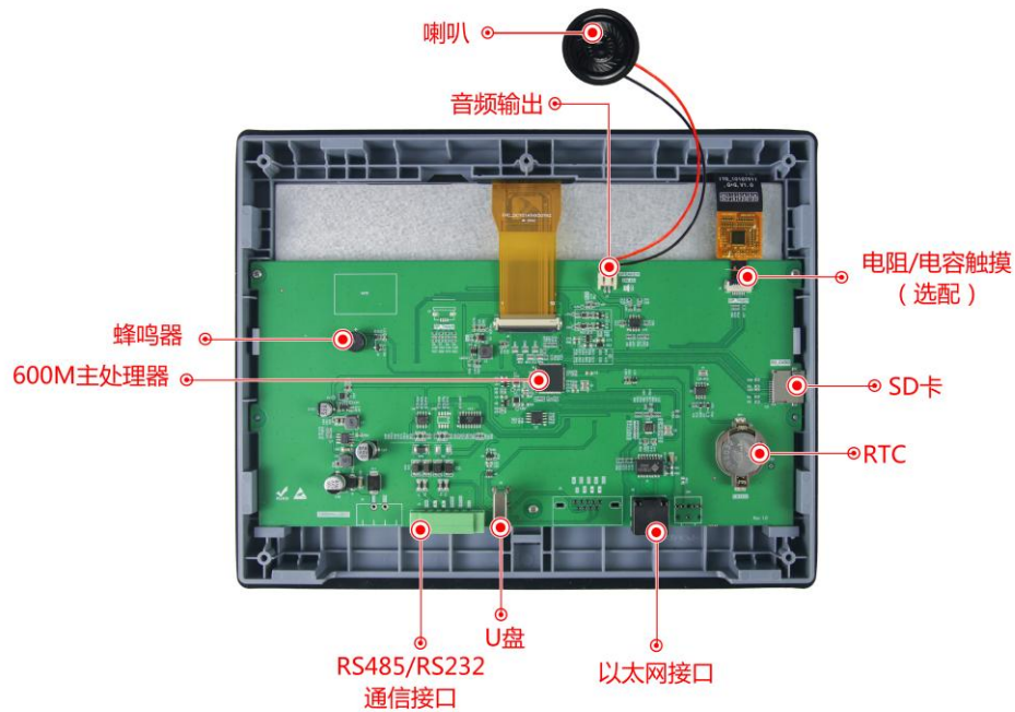
图 1-2 硬件配置图
